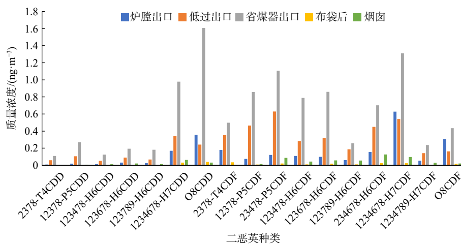
(a) 17种二恶英在不同采样点的质量浓度
