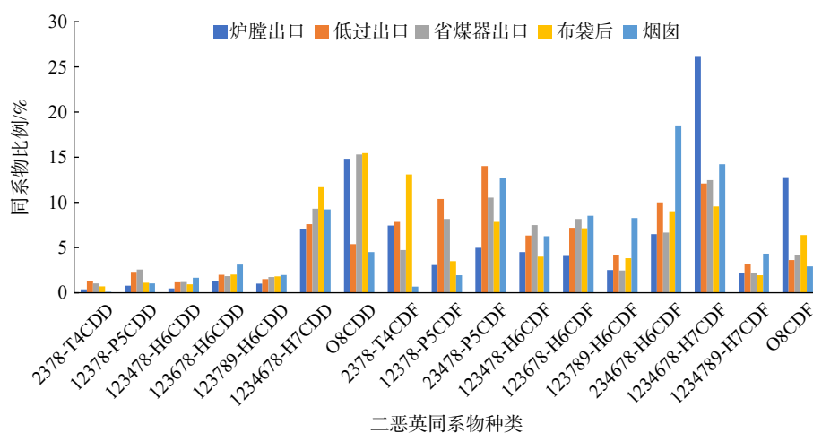
(b) 17种二恶英同系物在不同采样点的占比
